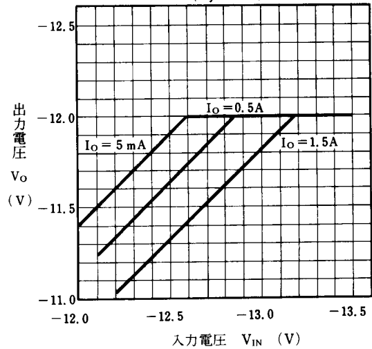
NJM7900 シリーズ保護回路動作特性例 ( T_j = 25^\circ C )
