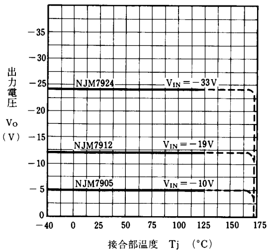
NJM7905/12/24 出力電圧温度特性例
