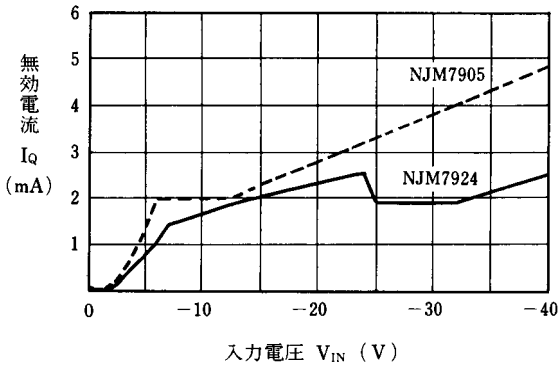
NJM7905/24 無効電流特性例 ( I_o = 0\text{ mA} , T_j = 25^\circ\text{C} )
