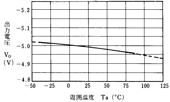
NJM7905 出力電圧温度特性例
