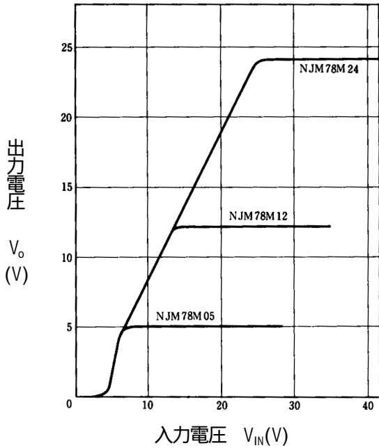
NJM78M05/M12/M24 出力電圧特性例 ( I_o = 350\text{mA} , T_j = 25^\circ\text{C} )
