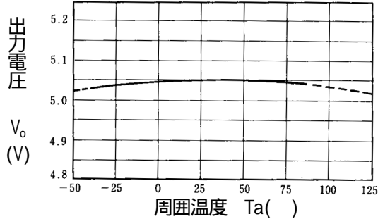
NJM78M05 出力電圧温度特性例
