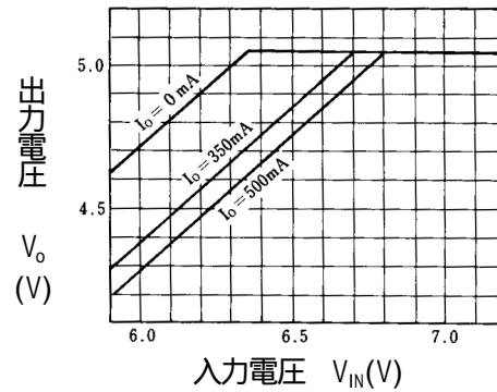
NJM78M05 入出力間電位差特性例 ( T_j = 25 )
