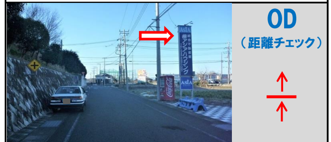
4図 右手の看板「アジアハウジング」 SCP~OD間の試走車の計測距離は 5.560 km
