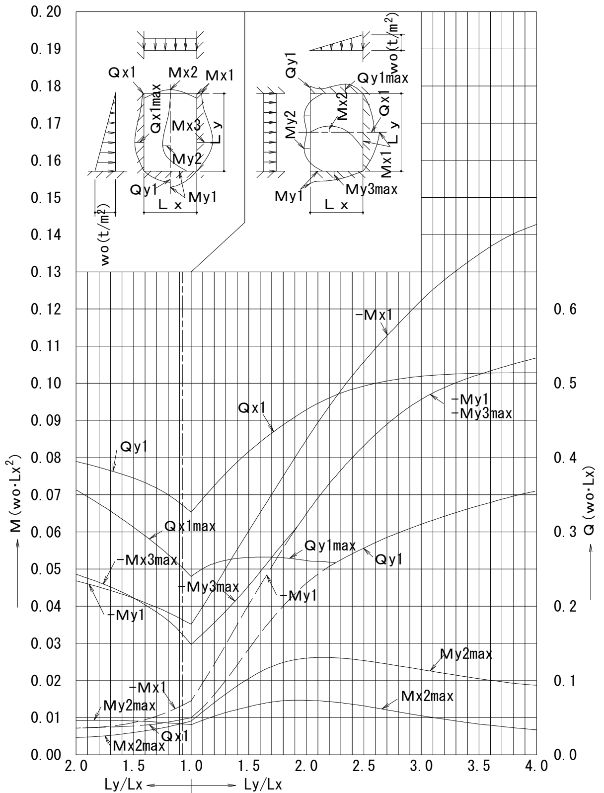
等変分布荷重時3辺固定1辺自由スラブの応力図
