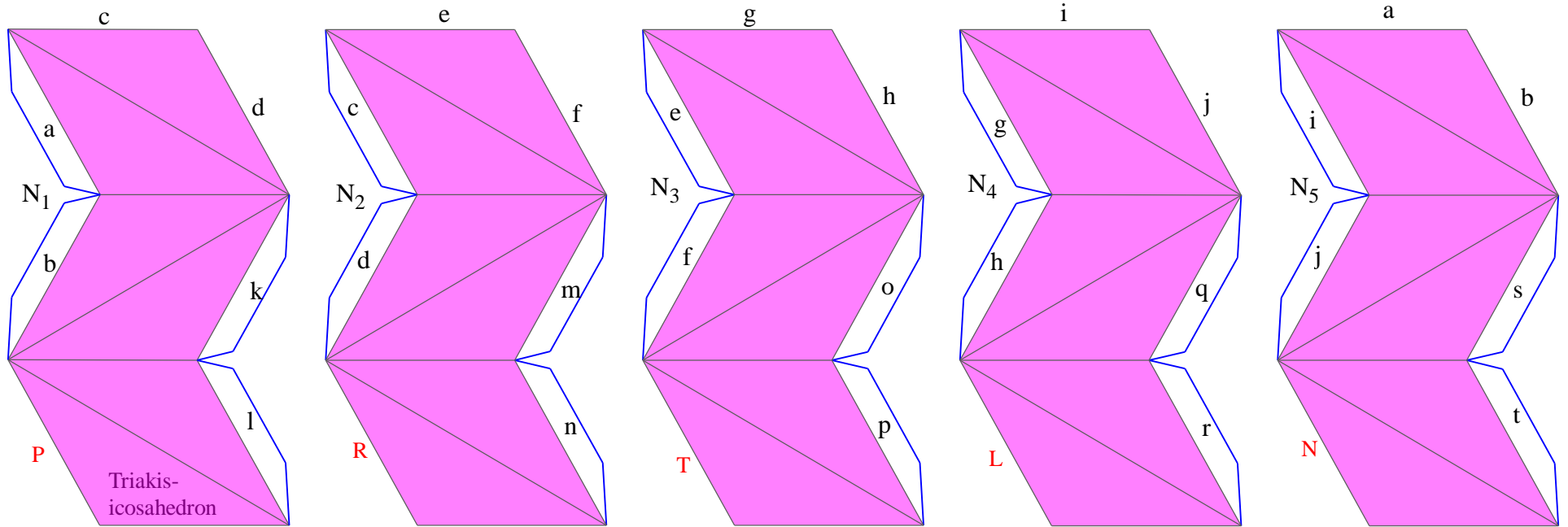
[3,10,10] 三方二十面体 Triakisicosahedron = 切頂十二面体の双対 改訂版2015.1.10
