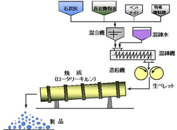
石炭灰人工骨材の製造法(特許第3280647号)
