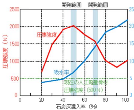
石炭灰と頁岩微粉末を混合による圧壊強度
