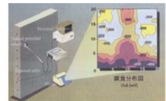
鉄筋腐食診断システム
