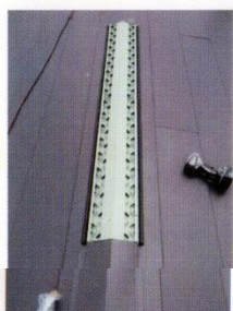
▲換気棟を付けます。
