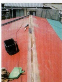
▲防水シートを張ります。
